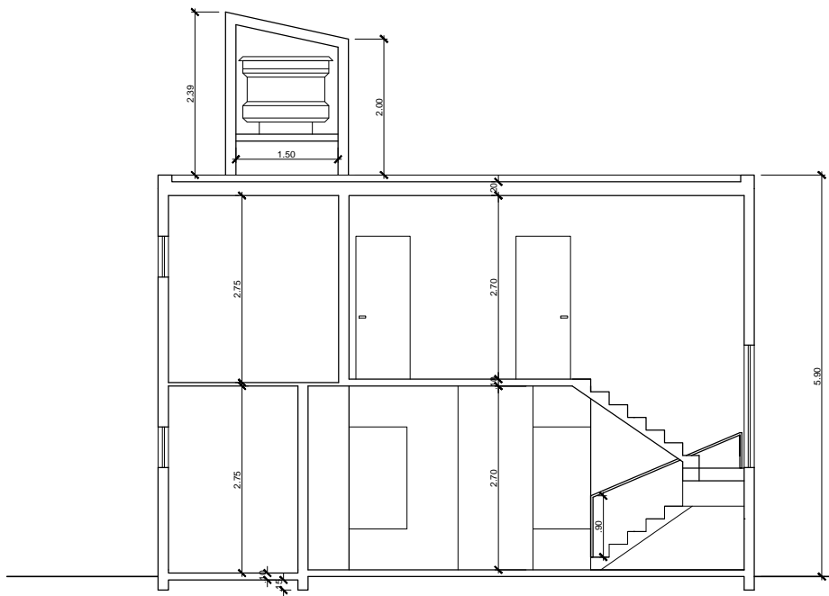
CORTE 1 ESC. 1/100
