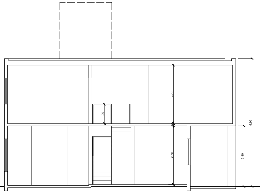
CORTE 2 ESC. 1/100
